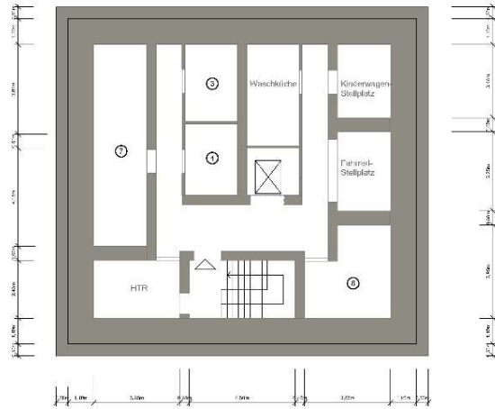
Grundriss UG 2 M 1:100
