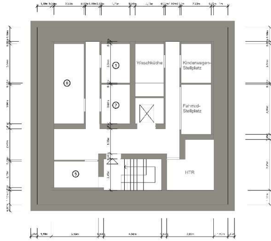
Grundriss UG 1 M 1:100
