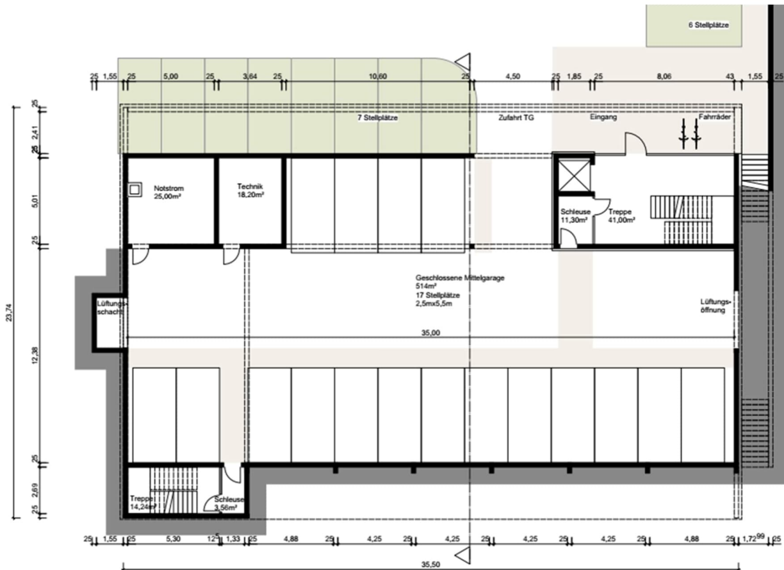
Entwurfsplanung - Untergeschoss
