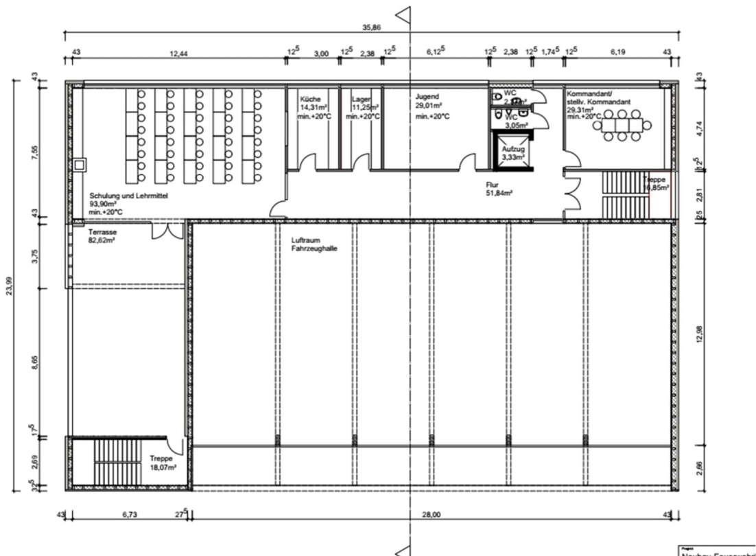
Entwurfsplanung - Obergeschoss
