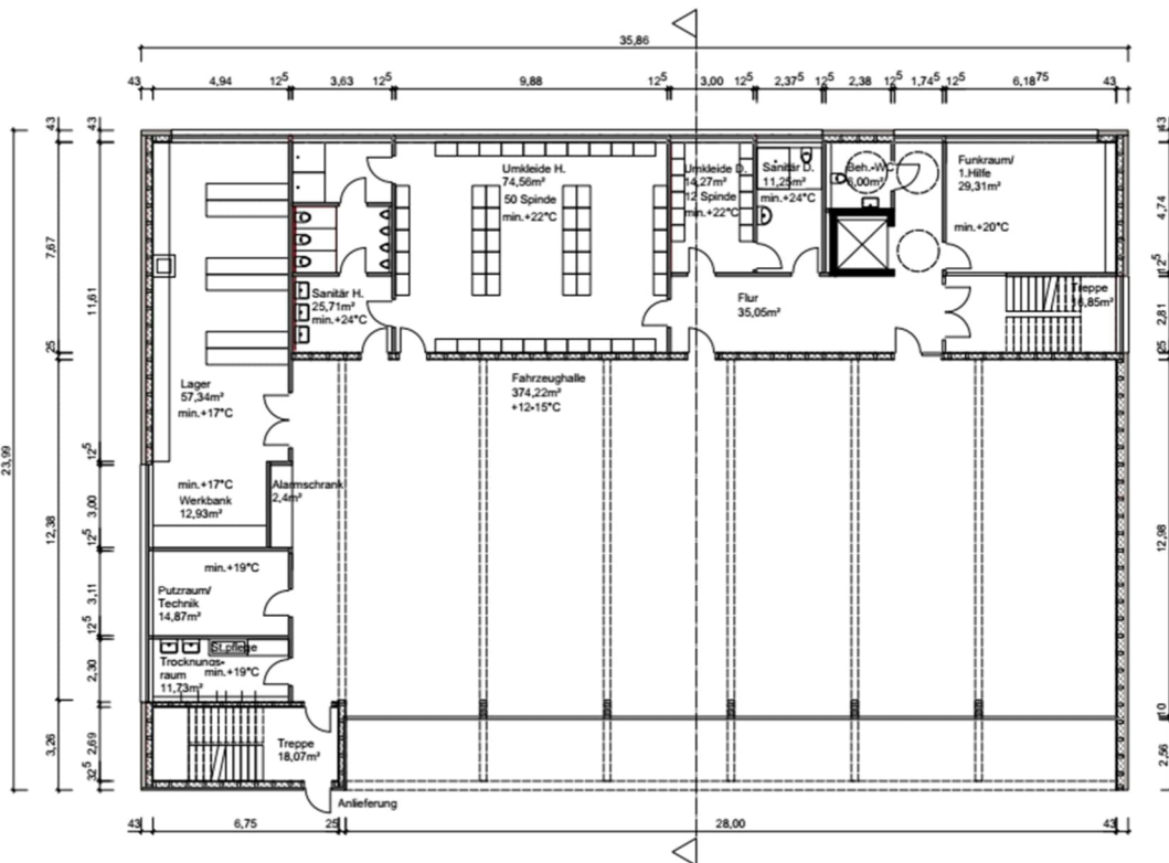
Entwurfsplanung - Erdgeschoss
