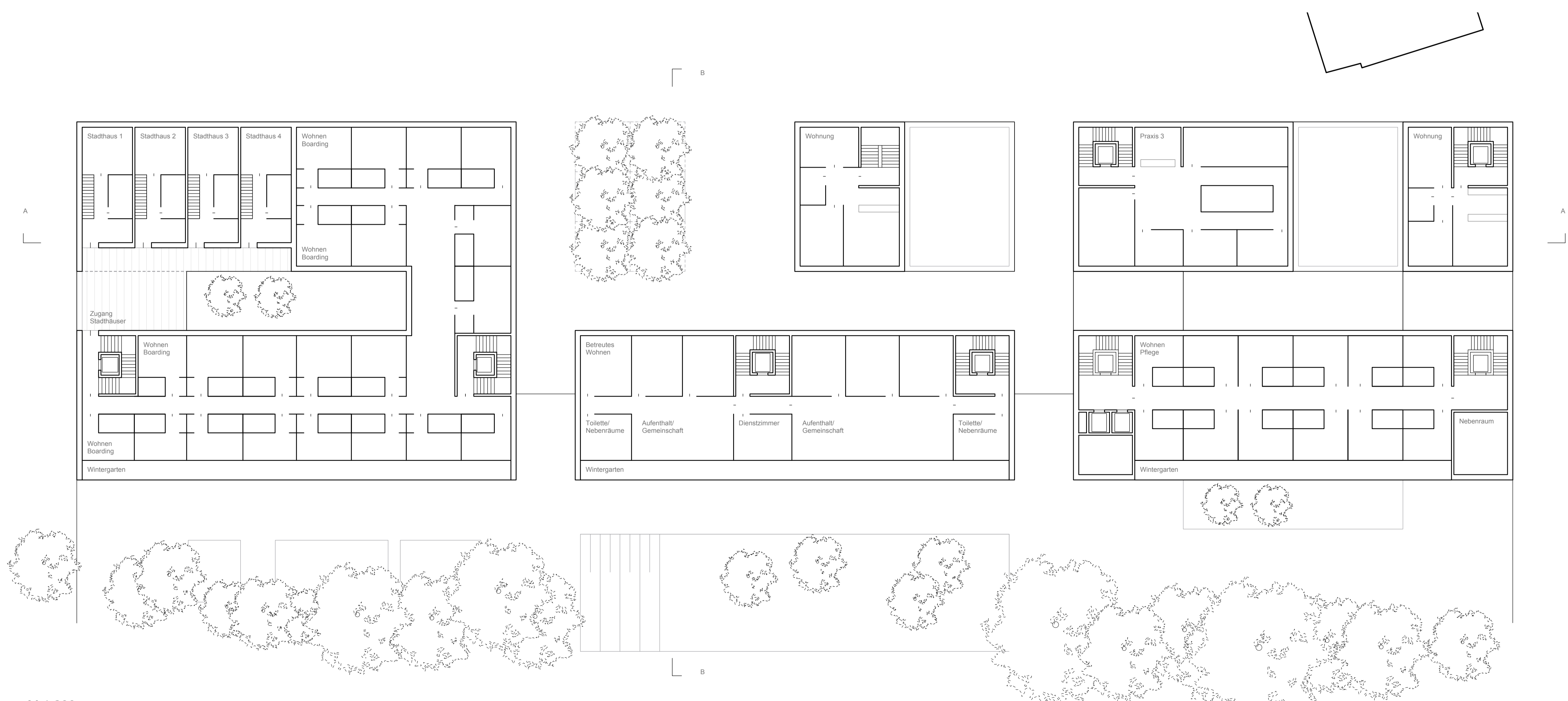
Grundriss 2. Obergeschoss M 1:200
